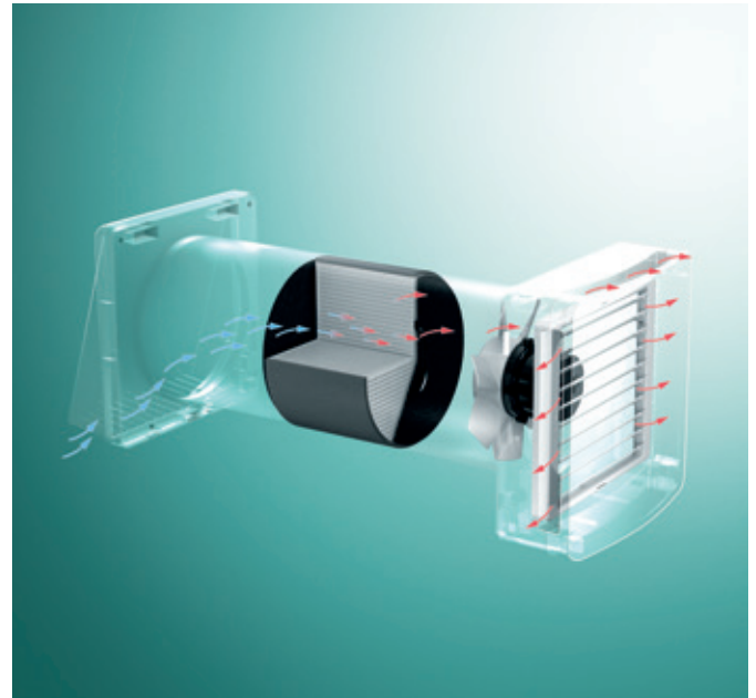
Dezentrale Lüftung recoVAIR 60 mit Wärmerückgewinnung
