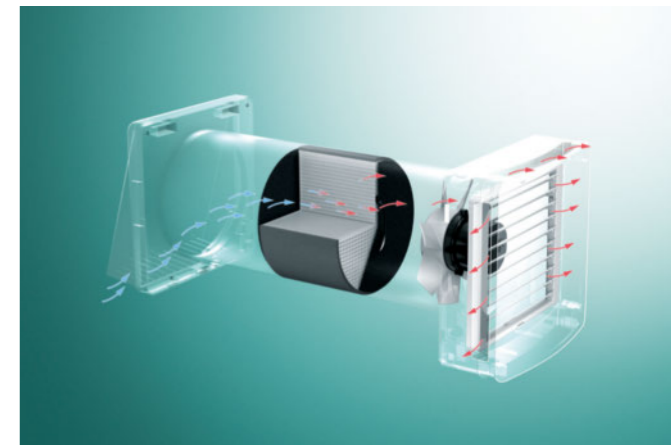
Dezentrale Lüftung recoVAIR 60 mit Wärmerückgewinnung
